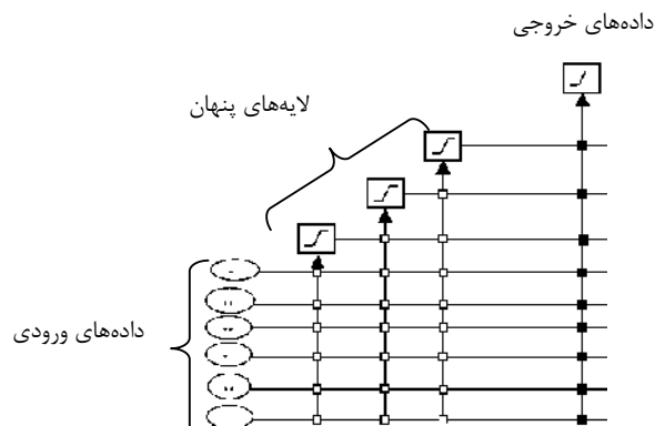
شکل ۴. ساختار شبکه آبشاری پس‌انتشار با سه لایه پنهان
