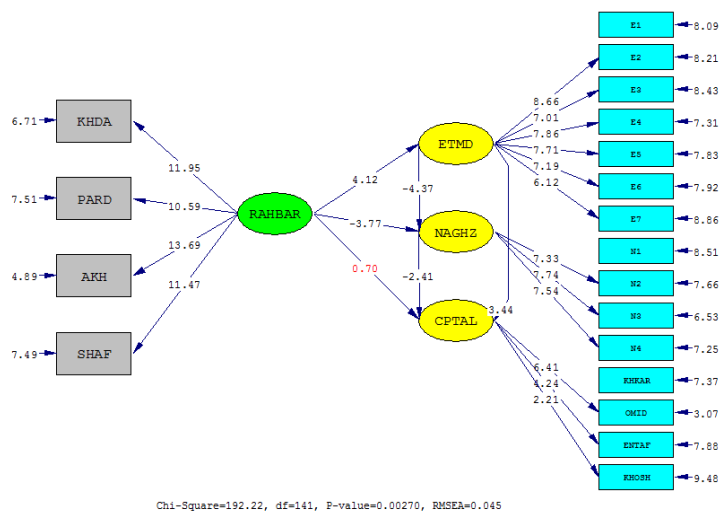
شکل ۲. مدل معالات ساختاری در حالت اعداد معناداری
