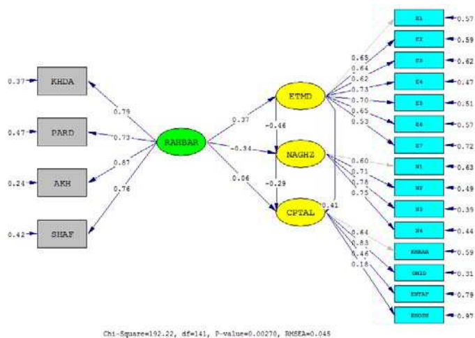
شکل ۱. مدل معالات ساختاری در حالت تخمین استاندارد
