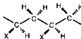
meso diad
