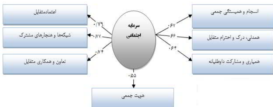
شکل ۱. مدل مفهومی
